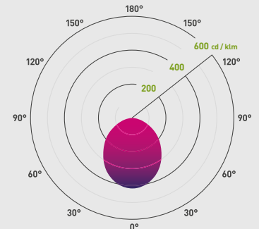
4000K 100° Weitere Diagramme finden Sie auf collingwoodlighting.com
