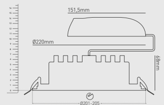
4000K 100° Weitere Diagramme finden Sie auf collingwoodlighting.com
